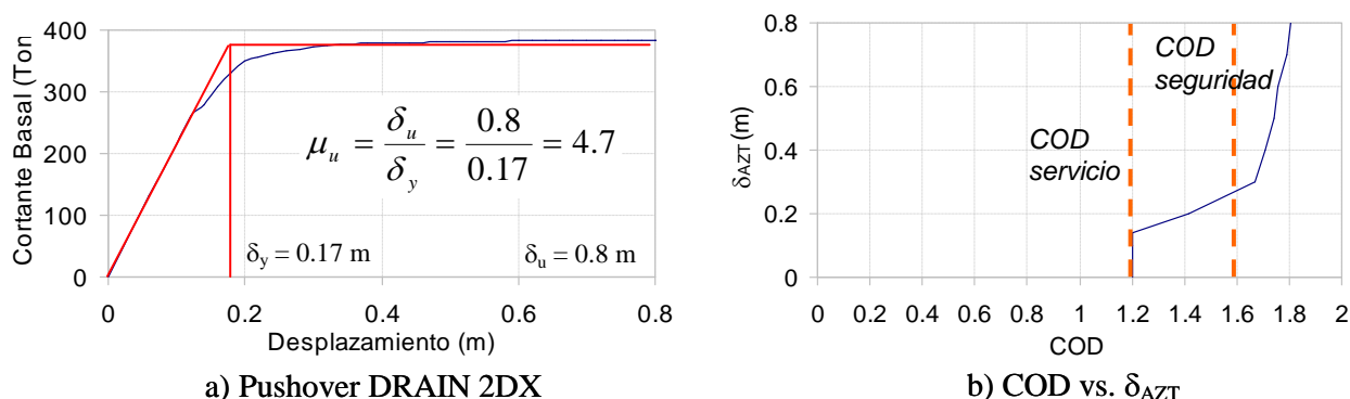
Figura 7. Comportamiento del edificio de 12 pisos en función de su desplazamiento de azotea
