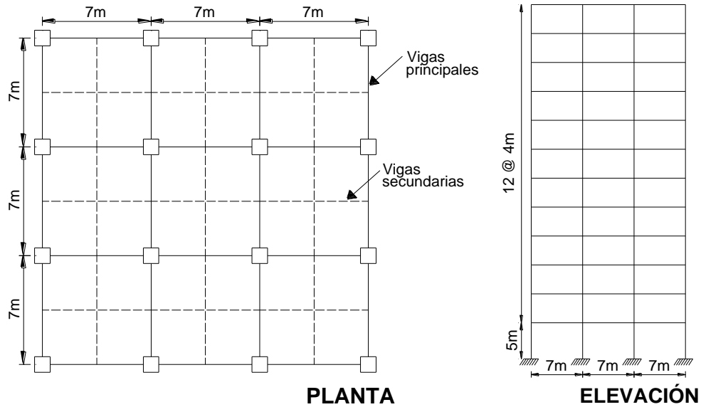
Figura 2. Planta y elevación del edificio
