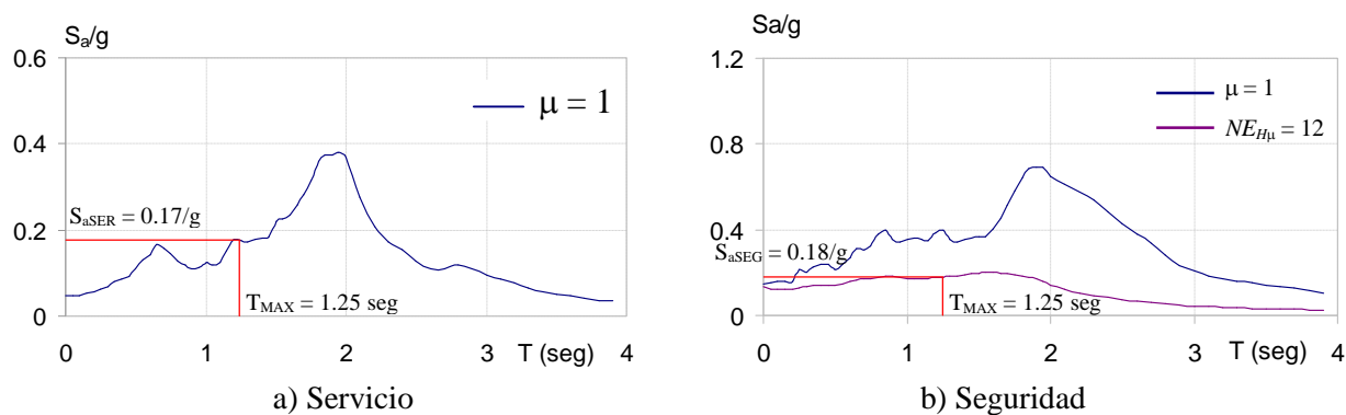
Figura 6. Determinación del cortante basal para servicio y seguridad
